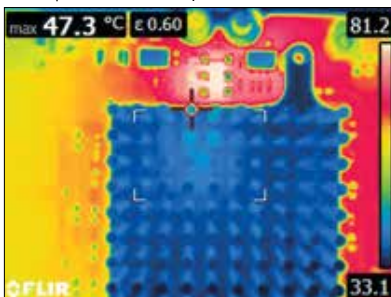
Erkennen Sie, wo Sie Wärmemanagement-Vorrichtungen hinzufügen müssen oder weglassen können
