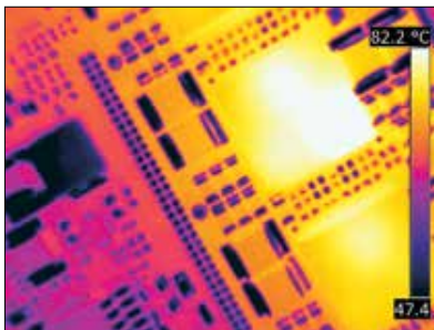
Messen Sie kleine Komponenten mit einem bis zu 170 µm kleinen Punkt pro Pixel
